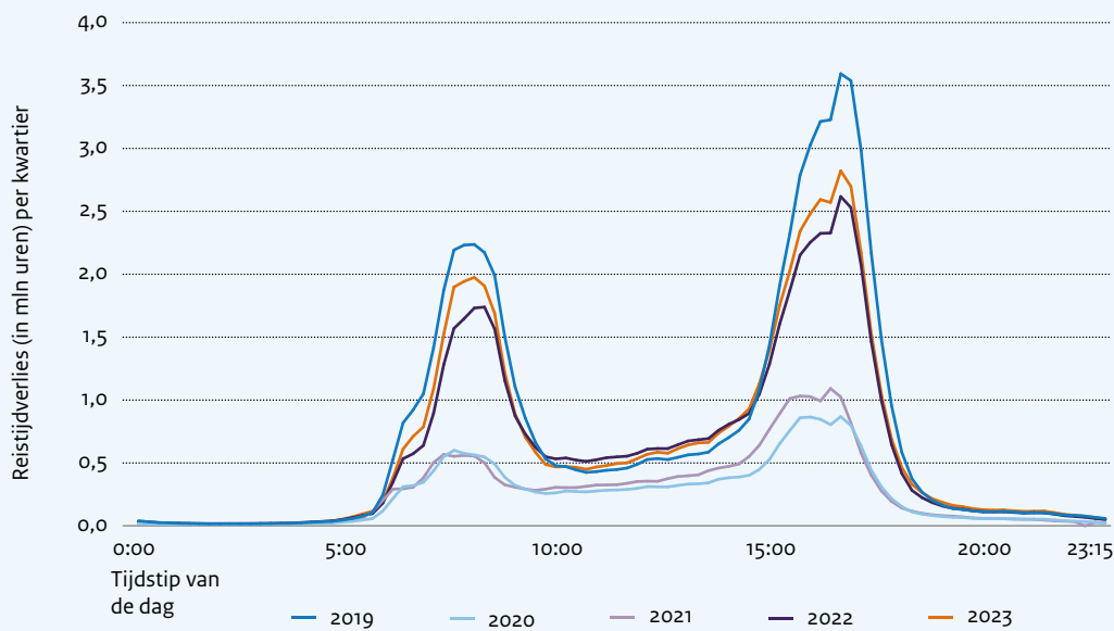
Figuur 4.4 Verdeling van het reistijdverlies per kwartier op het hoofdwegennet over de dag, 2019-2023
