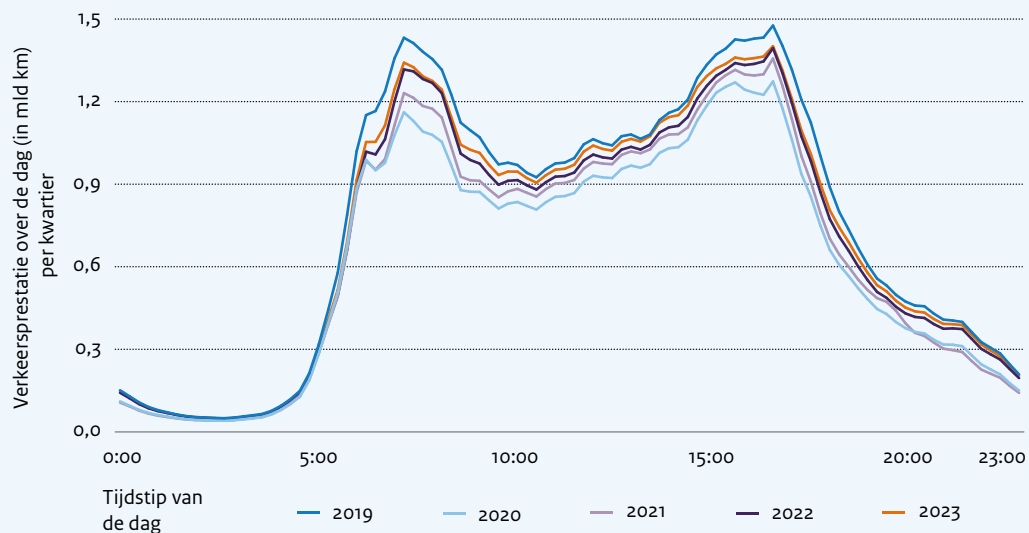
Figuur 4.2 Verdeling van de verkeersprestaties per kwartier op het hoofdwegennet over de dag, 2019-2023
